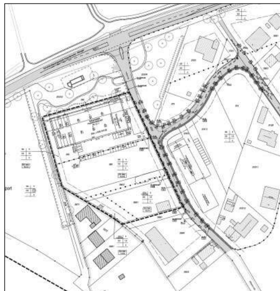
(nichtmaßstäblicher Lageplan)
